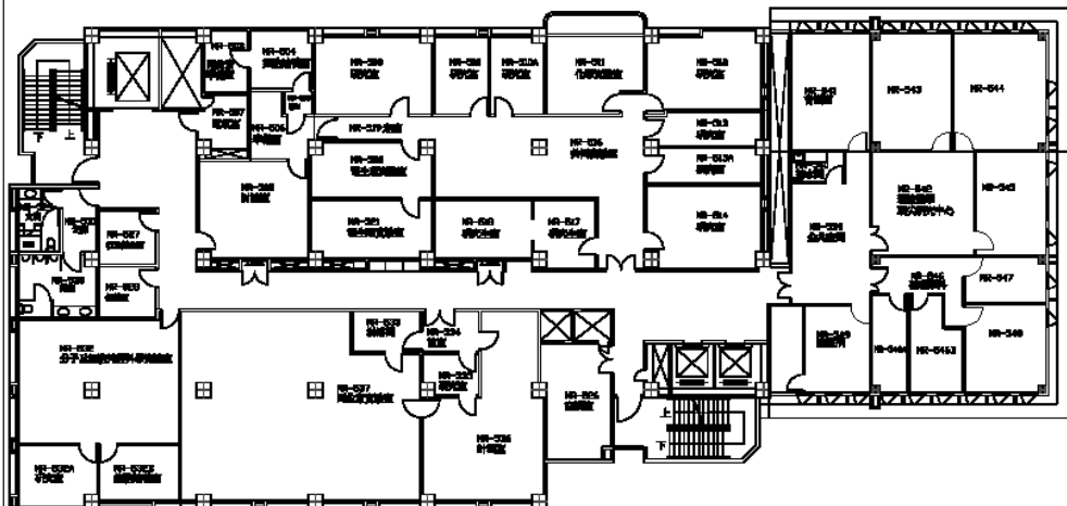
醫學研究大樓5F
