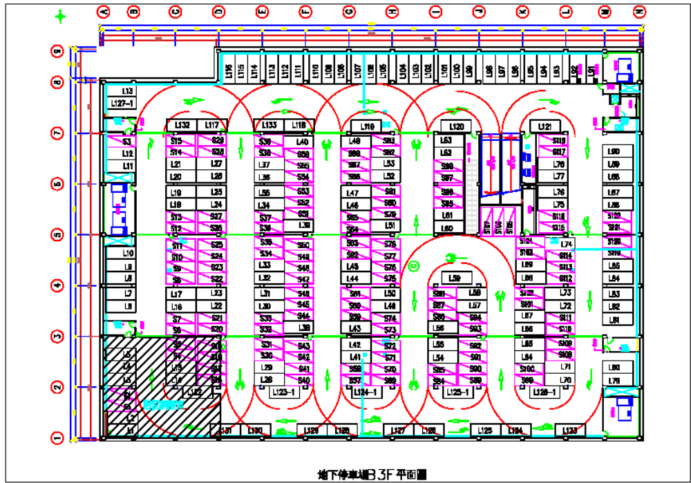
地下停車場3F平面圖
