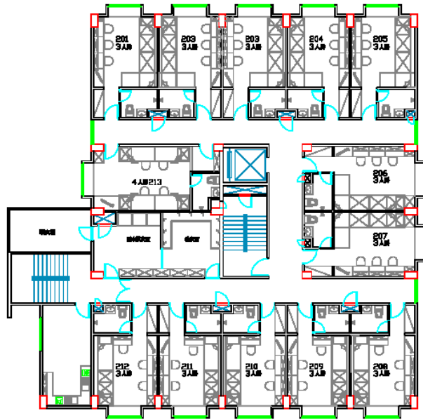
醫護宿舍二樓平面圖
