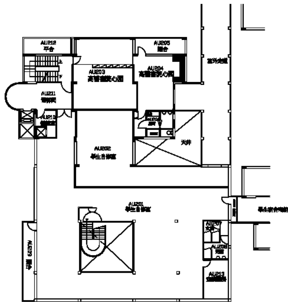
校友會館 二樓平面圖
