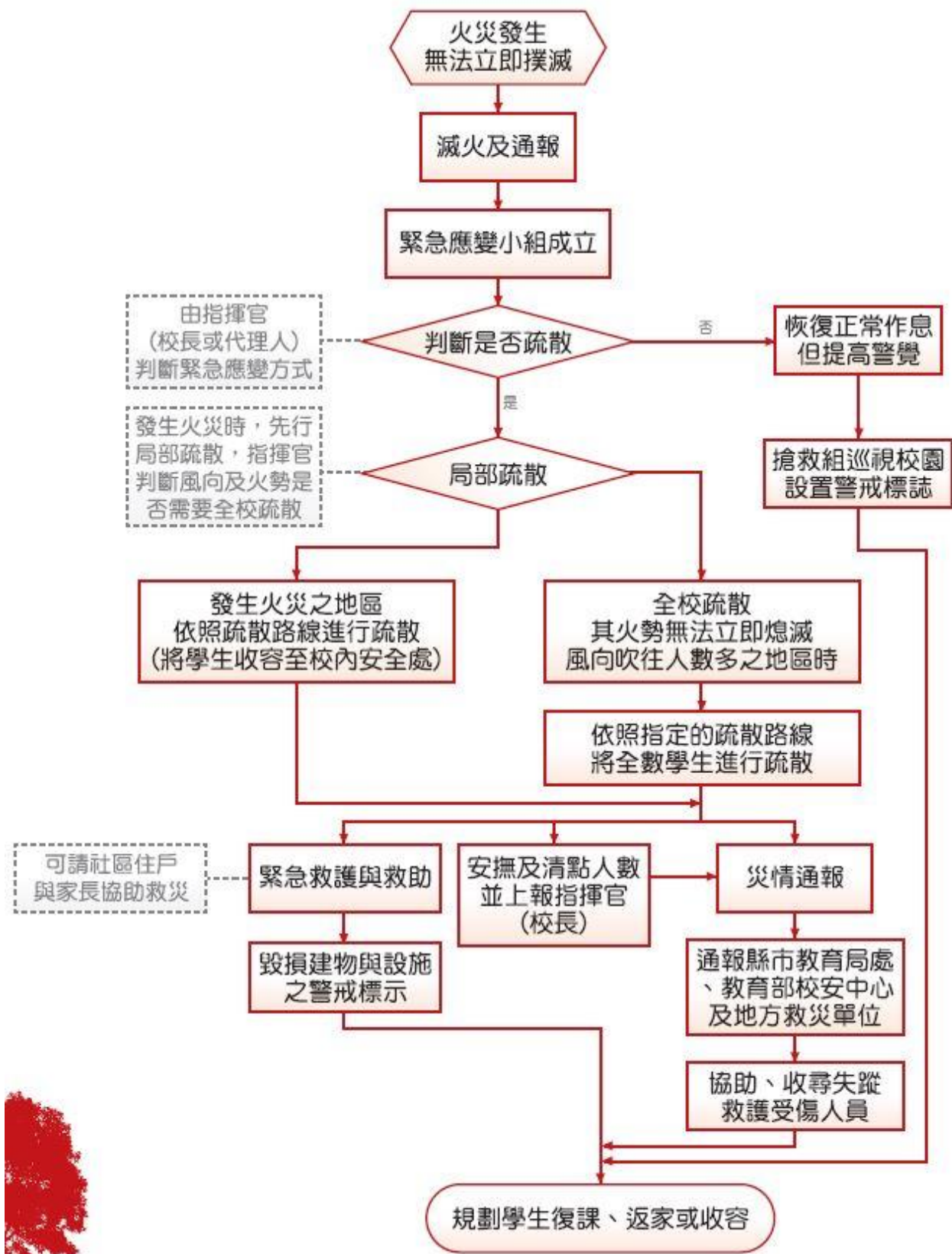
圖 8-1 火災災害應變工作流程圖
