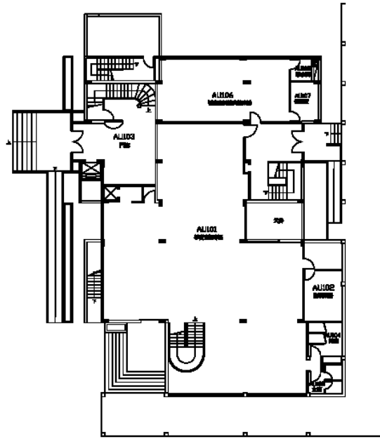
校友會館一樓平面圖
